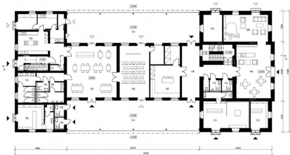
Pūdorys 1.NP
